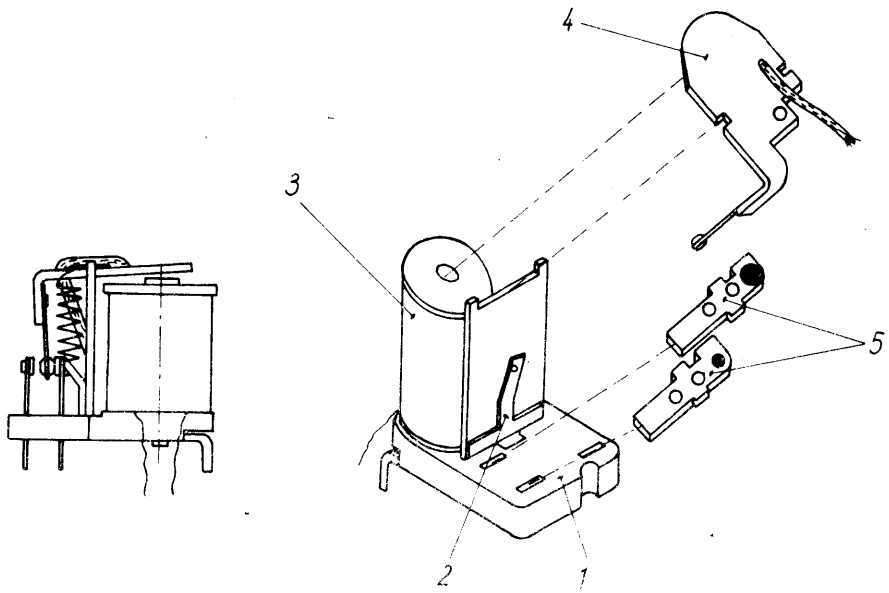
Montageanleitung für Relais
