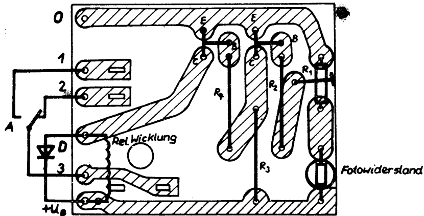
Bild 3: Ansicht der Leiterseite
