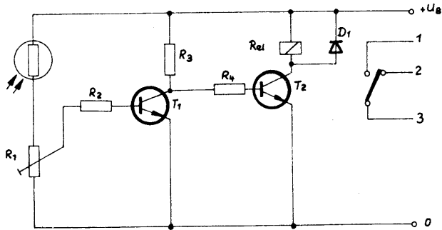
Bild 1: Lichtempfindlicher Schalterbaustein
