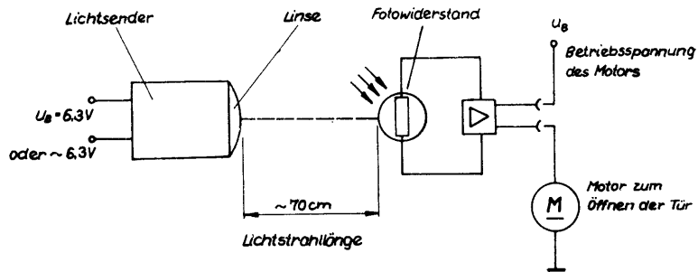
Bild 4 · Lichtschranke
